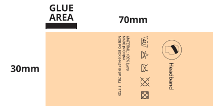
OPTIONAL - PAPER WRAPPING „B“ (SCALE 4:1)
